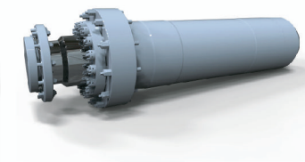
350吨压机油缸
